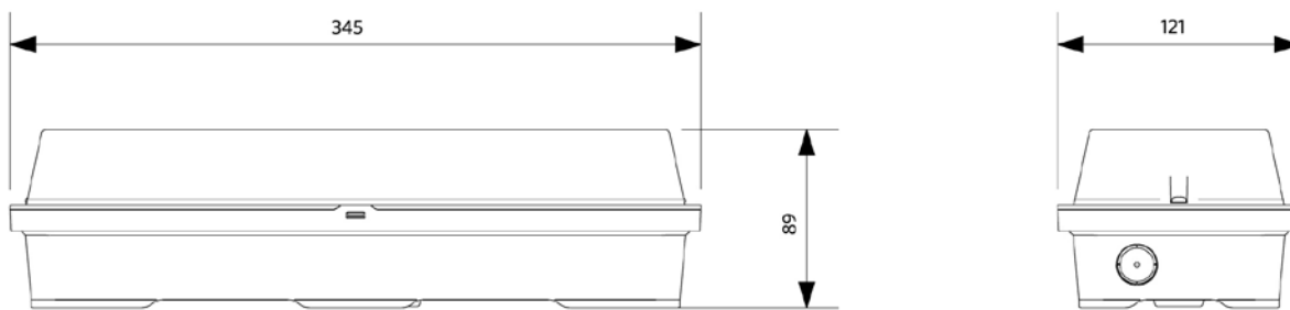
LEDPorch-E Re120
